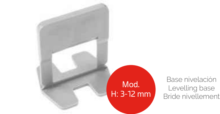
H: 3-12 MM BASE NIVELACIÓN Levelling base / Bride nivellement
