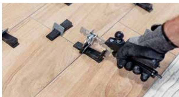
4. Apretar / Tighten / Serrer
